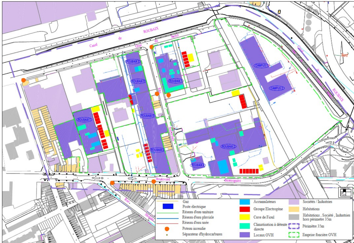
plan de l'installation 1/1000 (source : dossier).
